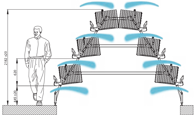
SuperTripleDeck para climas tropicales – el aire puede fluir sin dificultad a través del sistema
