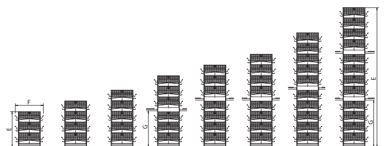
Sección transversal de jaula: UV 550, 600, 600-plus, 639, 788 sin conducto de aire
