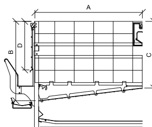
Клетка в разрезе: UV 550, 600, 600-plus, 639, 788 без воздушного канала
