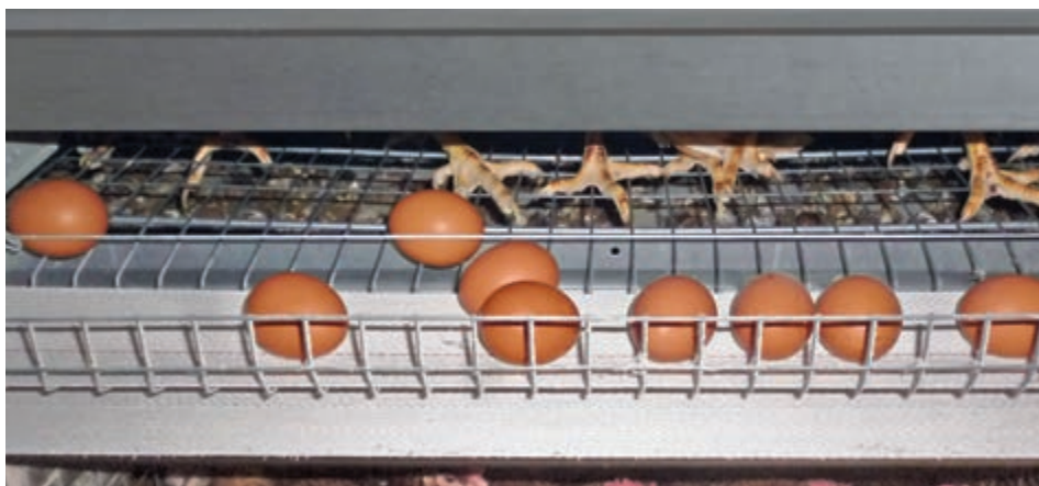
EggSaver опущен → мягкое притормаживание яйца
